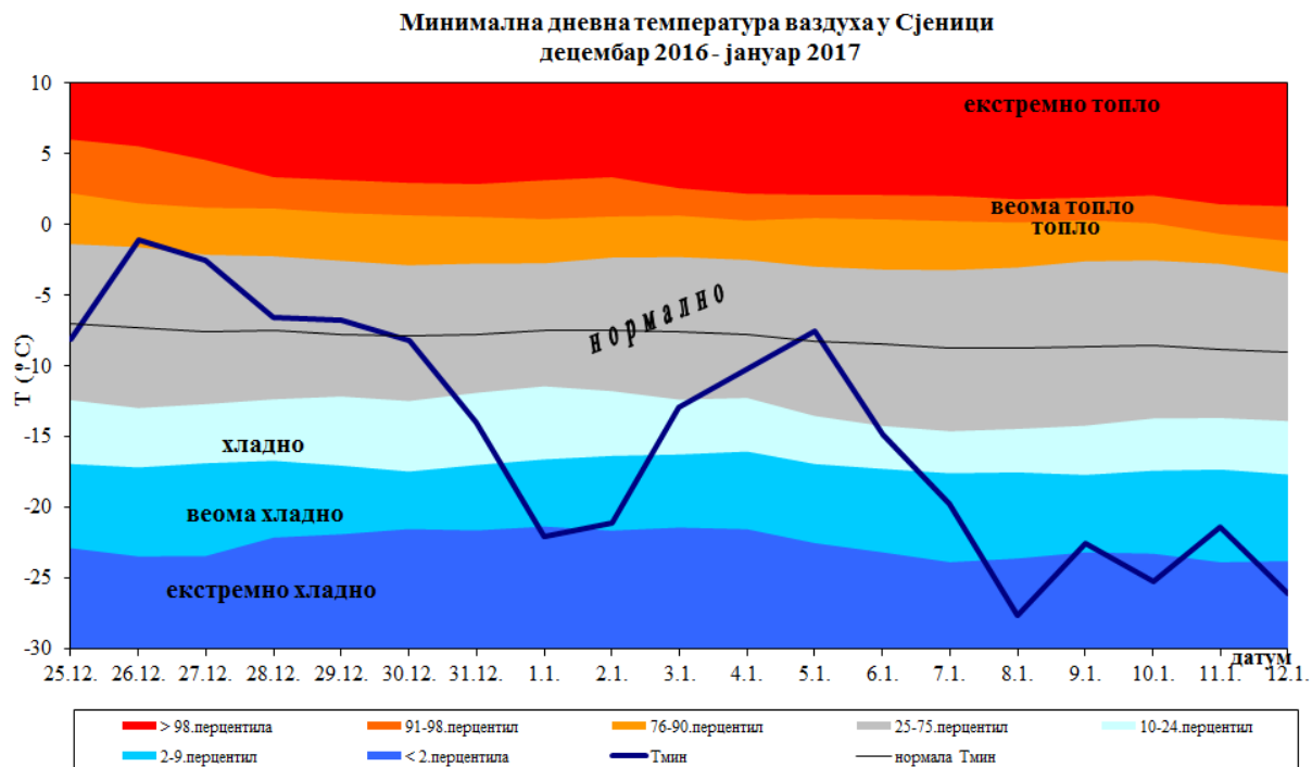
Слика 7. Минимална температура ваздуха у Сјеници за период од 25. децембра 2016. до 12. јануара 2017. године и припадајуће категорије према методи перцентила
