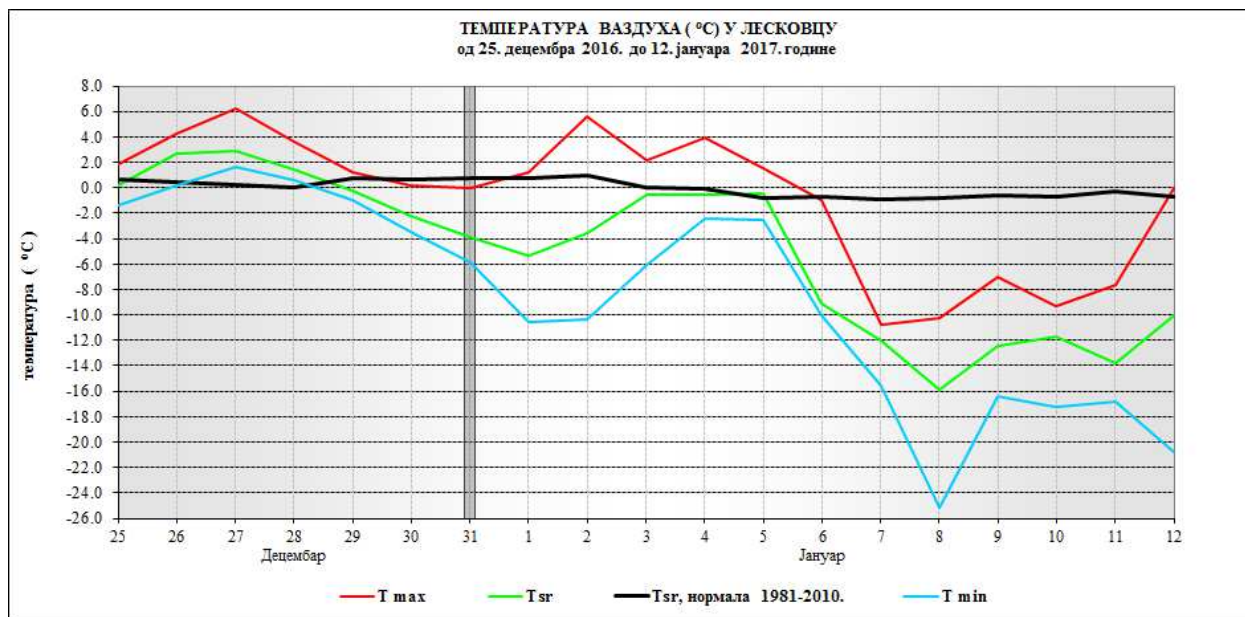
Слика 11. Средња, максимална и минимална температура ваздуха у Лесковцу, од 25. децембра 2016. до 12. јануара 2017. године, у односу на референтни период 1981-2010.
