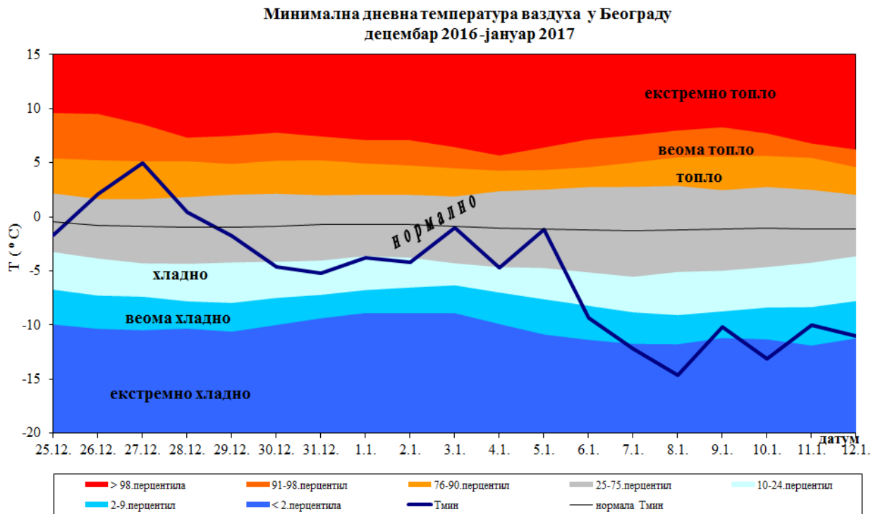
Слика 5. Минимална температура ваздуха у Београду за период од 25. децембра 2016. до 12. јануара 2017. године и припадајуће категорије према методи перцентила
