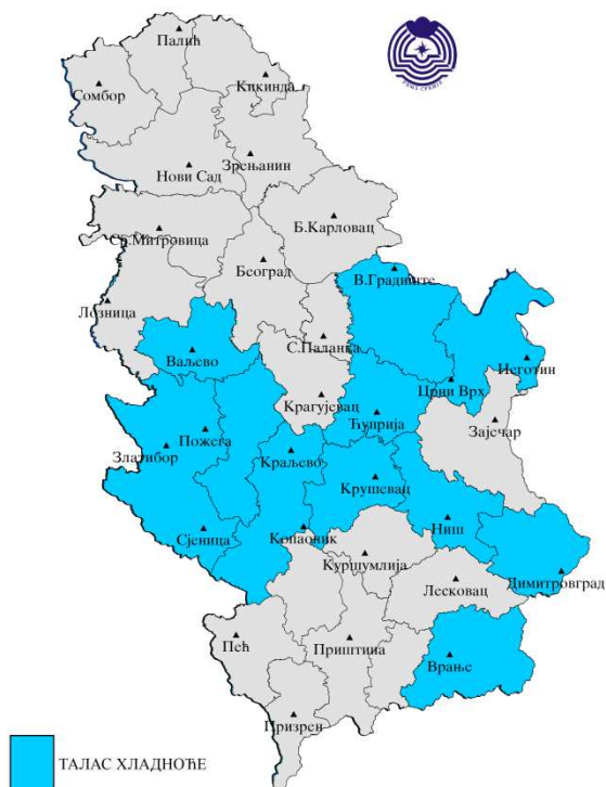
Окрузи у Србији захваћени таласом хладноће дана 13.1.2017.год.
