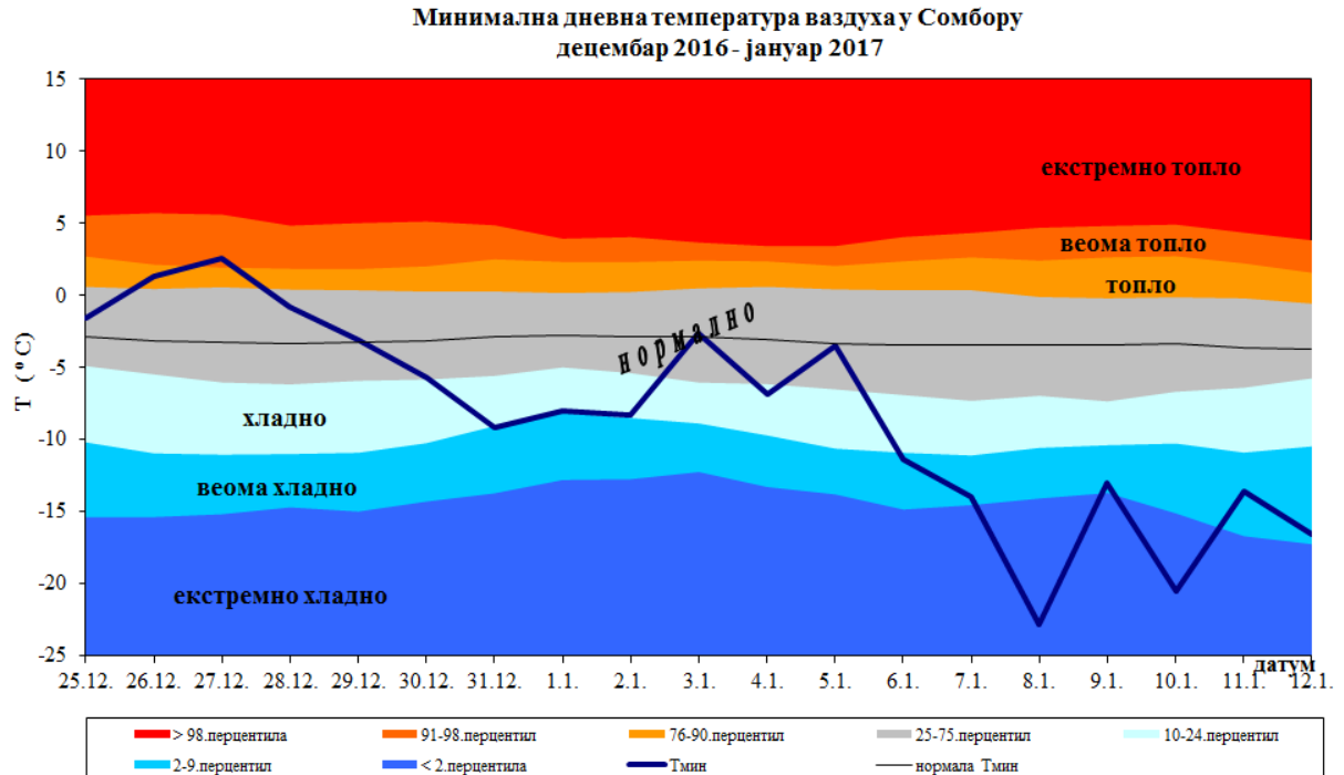
Слика 6. Минимална температура ваздуха у Сомбору за период од 25. децембра 2016. до 12. јануара 2017. године и припадајуће категорије према методи перцентила
