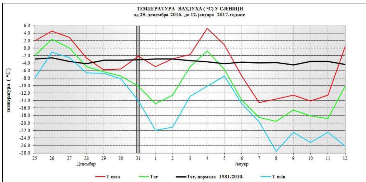
Слика 12. Средња, максимална и минимална температура ваздуха у Сјеници, од 25. децембра 2016. до 12. јануара 2017. године, у односу на референтни период 1981-2010.
