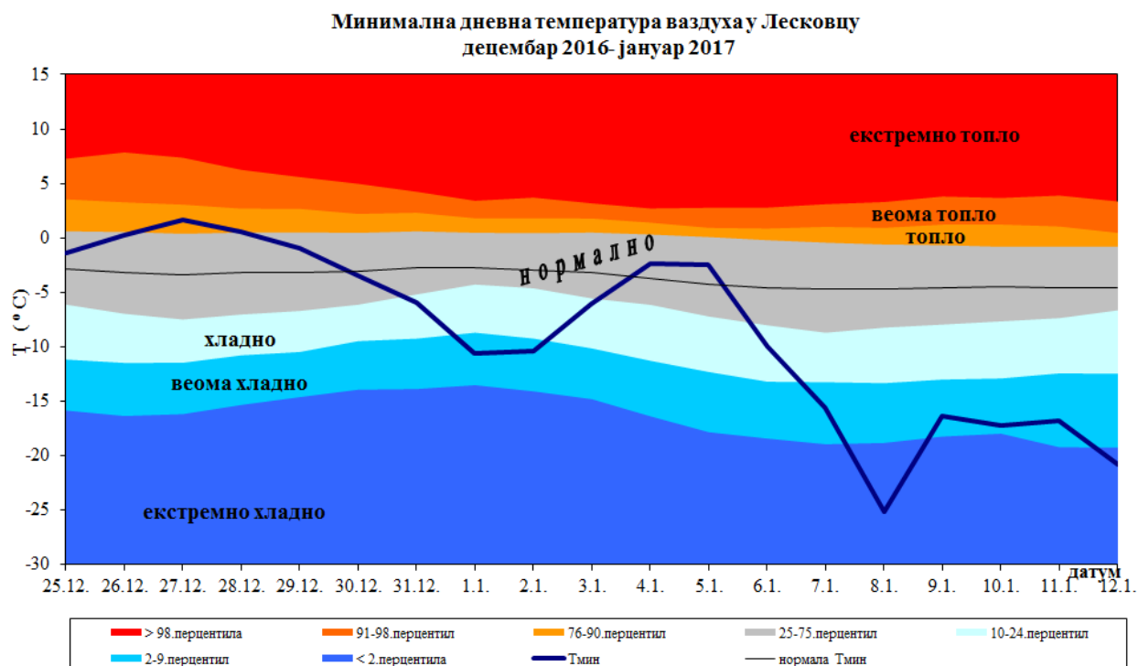
Слика 8. Минимална температура ваздуха у Лесковцу за период од 25. децембра 2016. до 12. јануара 2017. године и припадајуће категорије према методи перцентила
