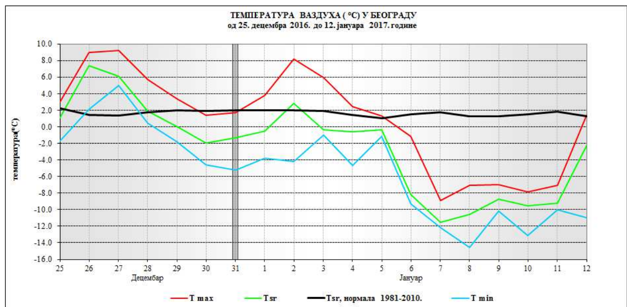
Слика 10. Средња, максимална и минимална температура вазуа у Београду, од 25. децембра 2016. до 12. јануара 2017. године, у односу на референтни период 1981-2010.
