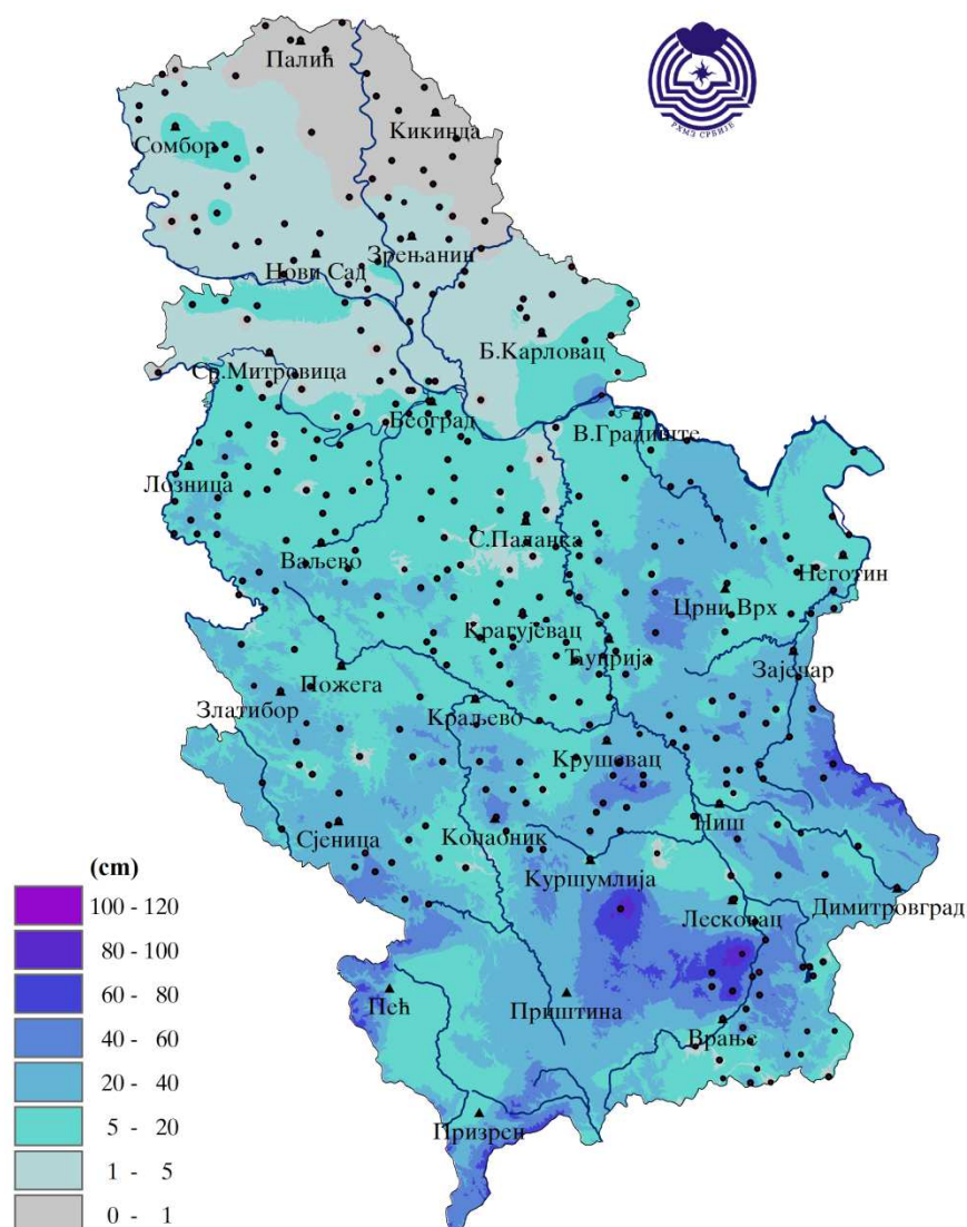
Слика 14. Просторна расподела максималне висине снежног покривача у Србији за 10. јануар 2017. године на основу података са 28 Главних метеоролошких станица, 51 климатолошке и 315 падавинских станица
