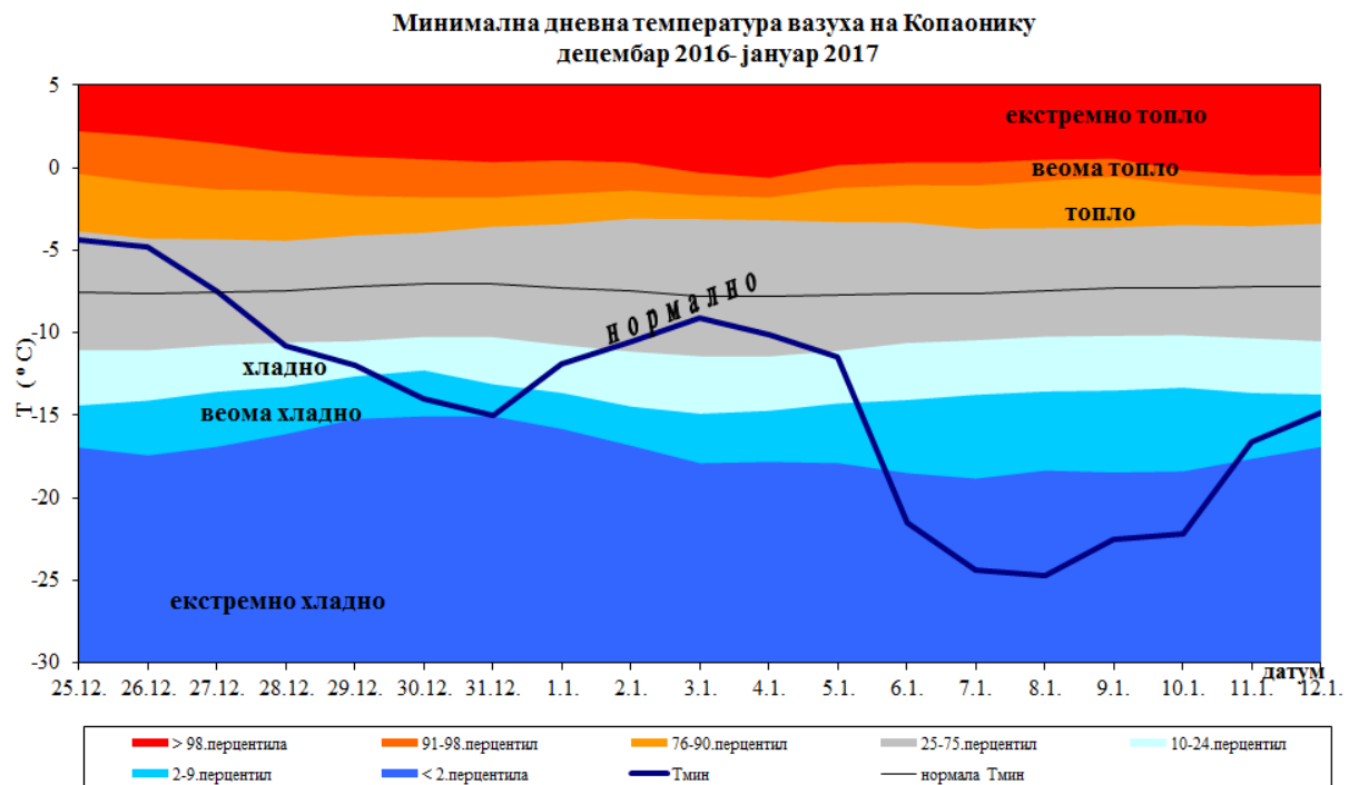
Слика 9. Минимална температура вазуа на Копаонику за период од 25. децембра 2016. до 12. јануара 2017. године и припадајуће категорије према методи перцентила
