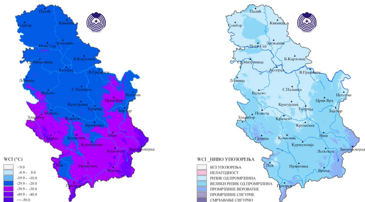
Слика 13. Просторна расподела минималне вредности WCI индекса за 8. јануар 2017. године (лево) и ниво упозорења (десно)
